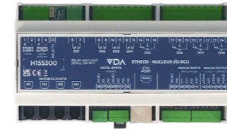
Etheos - Nucleus RCU ETHEOS CONTROLLER MODBUS
